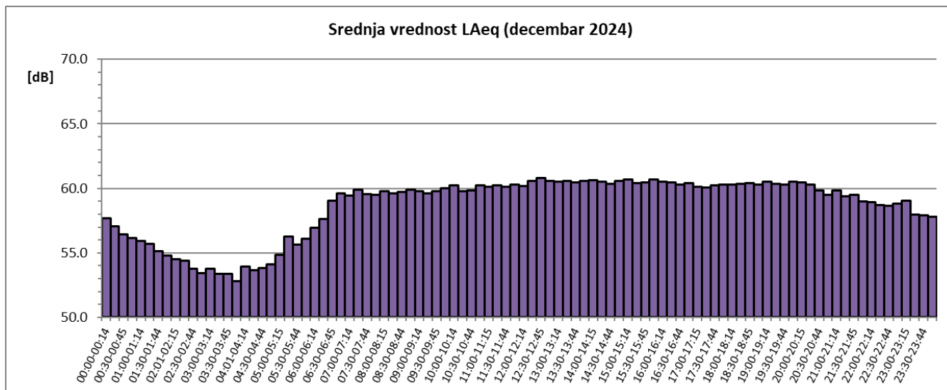
Sl. 3 Promene usrednjenih petnaestominutnih vrednosti ekvivalentnog nivoa buke u toku decembra 2024. za NMT-1
