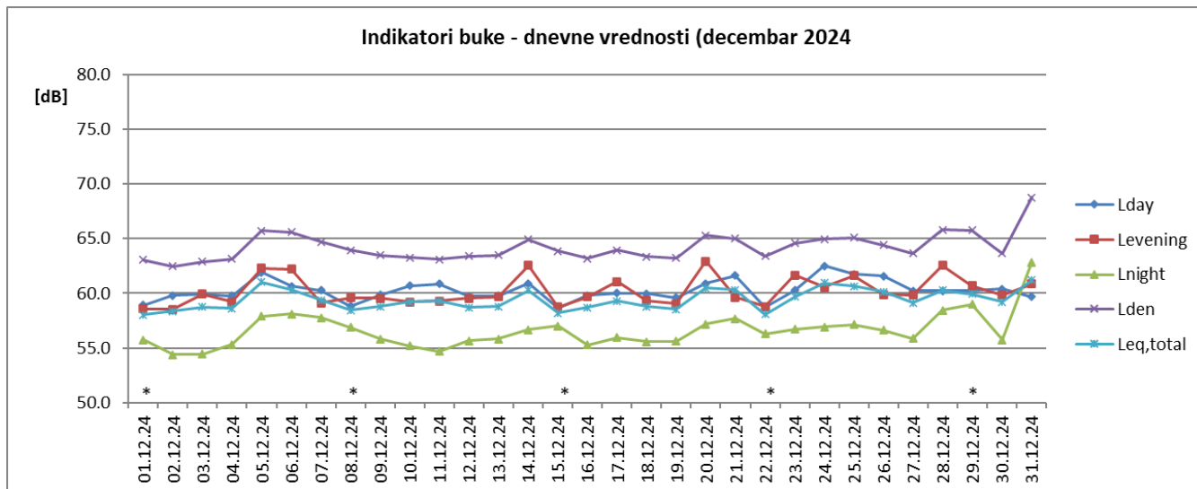
Sl. 1 Promene dnevnih vrednosti indikatora buke u toku decembra 2024. za NMT-1
