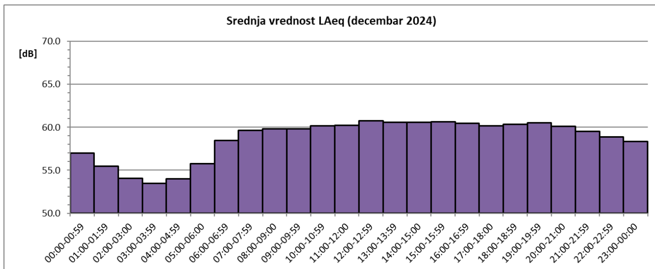
Sl. 2 Promene usrednjenih časovnih vrednosti ekvivalentnog nivoa buke u toku decembra 2024. za NMT-1
