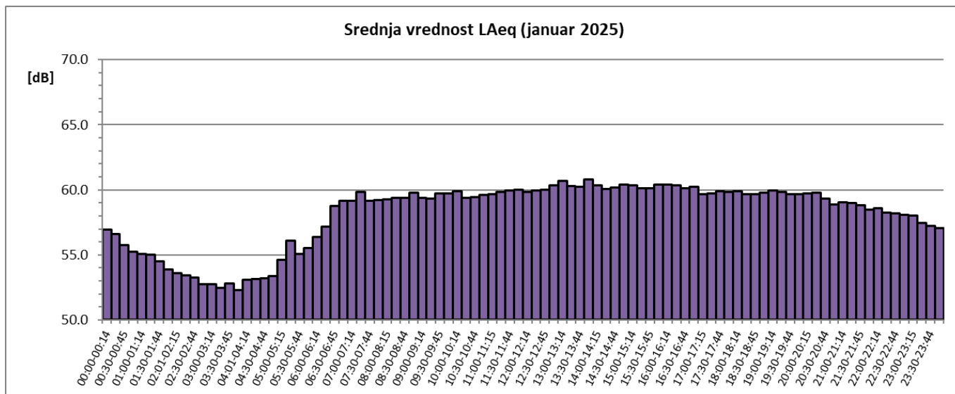
Sl. 3 Promene usrednjenih petnaestominutnih vrednosti ekvivalentnog nivoa buke u toku januara 2025. za NMT-1
