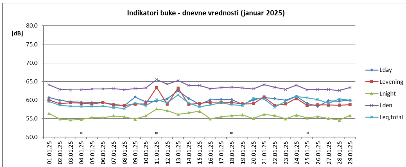
Sl. 1 Promene dnevnih vrednosti indikatora buke u toku januara 2025. za NMT-1
